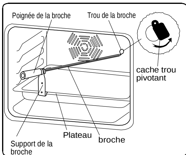
Modèle avec support sur plateau
