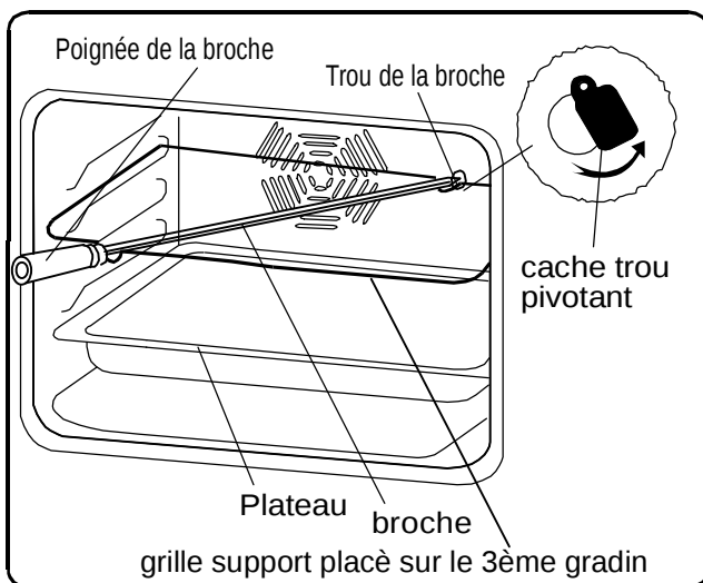
Modèle avec support sur grille
